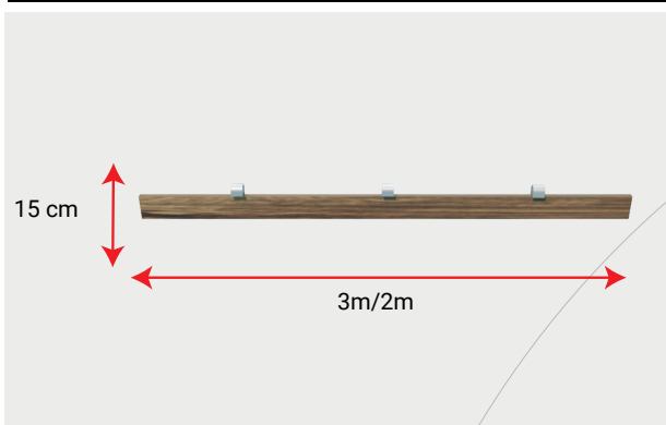
103/S250 - Kantplank
